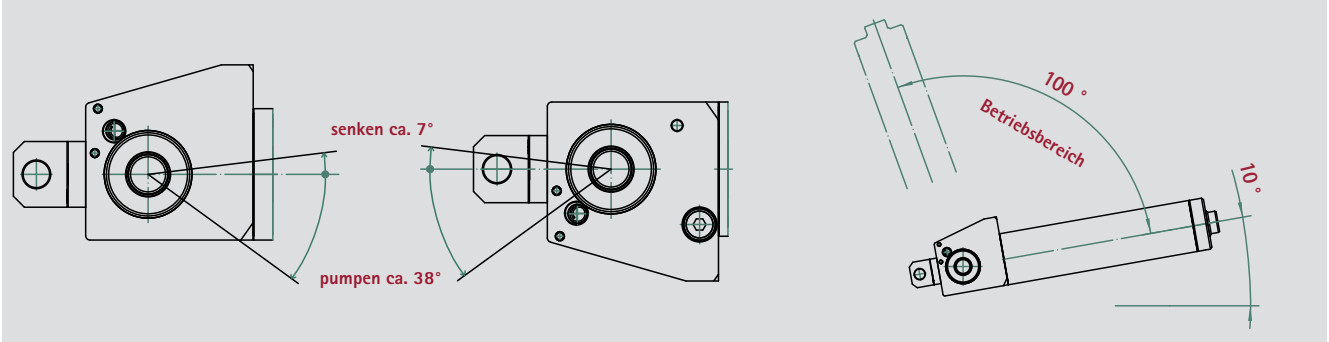
Einbaulage
