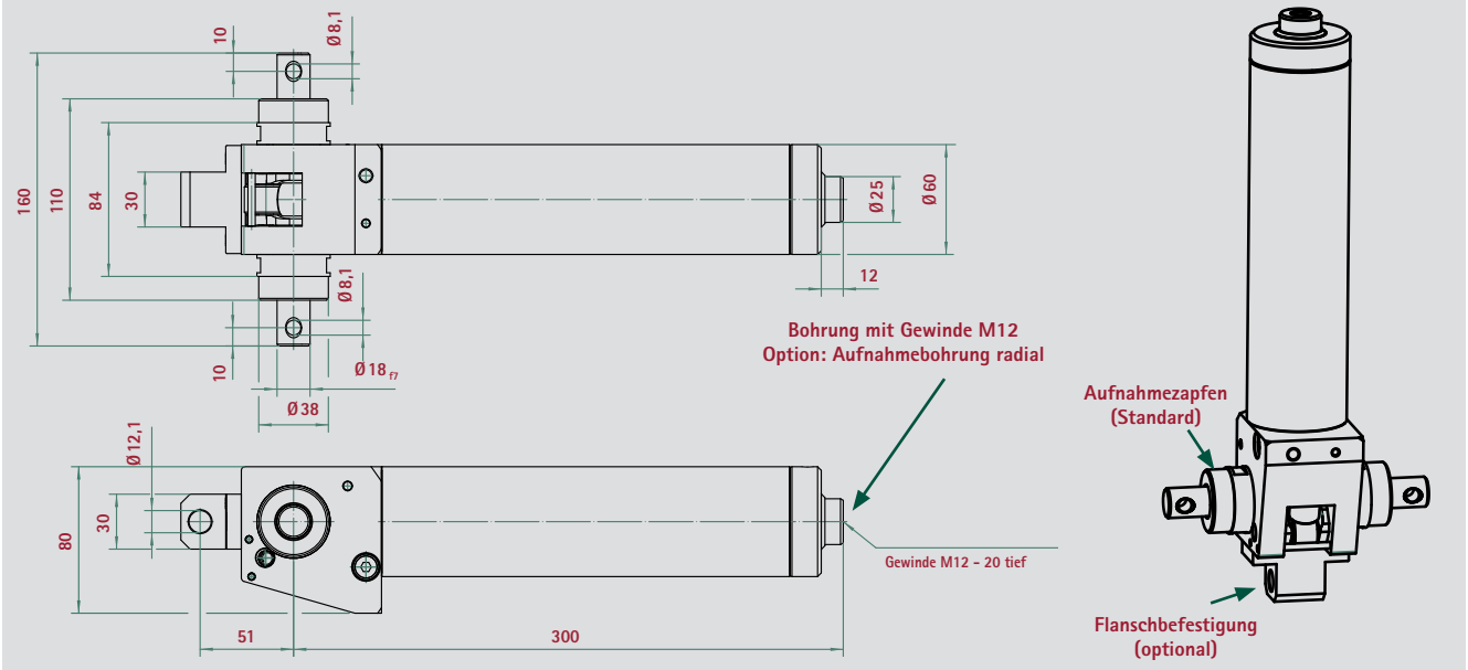
Baumaßreihe 2 am Beispiel Hub 200 mm
